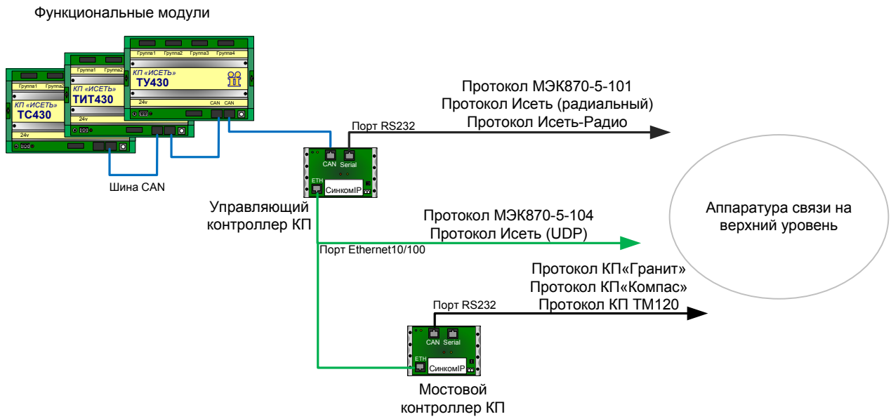
1. Типовая схема КП «Исеть» с мостовым контроллером связи
