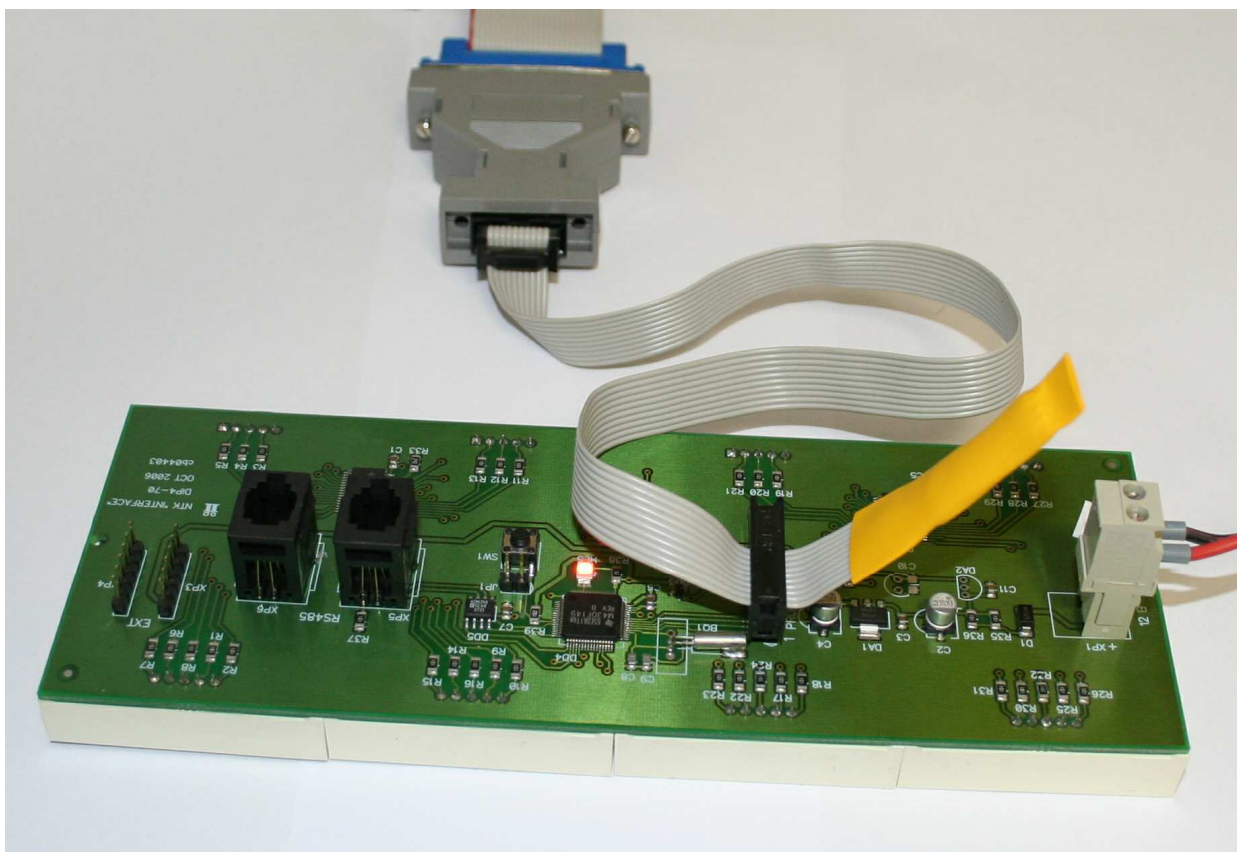
Подключение программатора к индикатору
