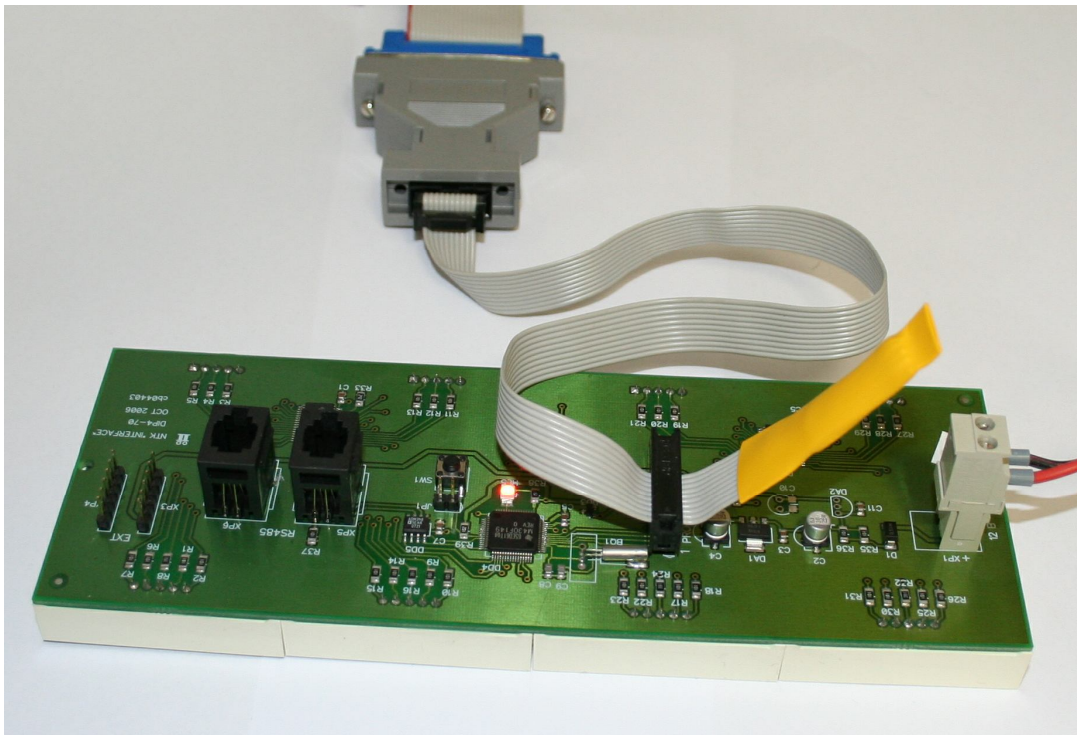
Подключение программатора к индикатору
